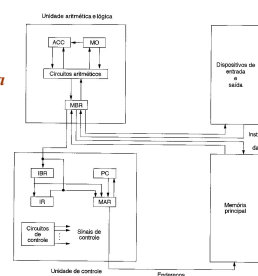
Figura 1.11 Diagrama em bloco da estrutura do IAS.
