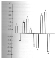
Figura 1.4 Exemplo de representação de 10 algarismos por níveis de tensão diferentes, em míquias decimais.
